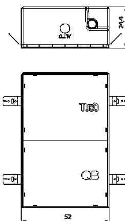
Ingombri predisposizione nuova QB ad incasso
