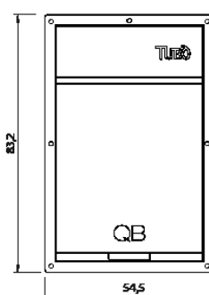
Ingombri nuova QB ad incasso completa
